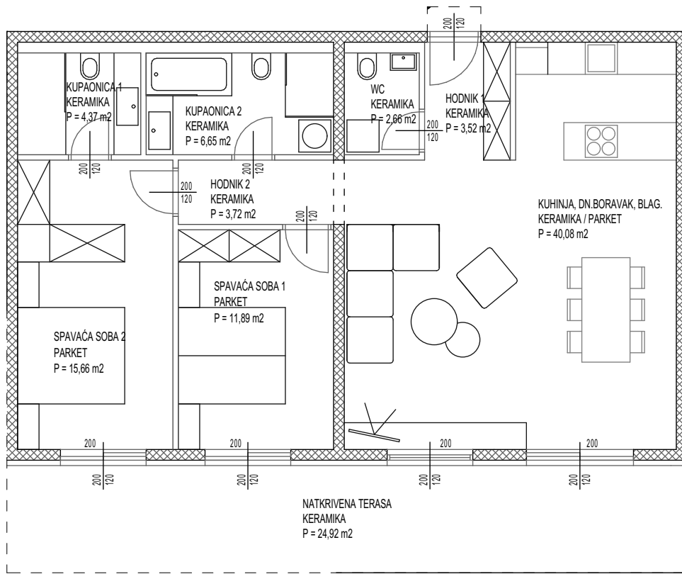
Tlocrt stana
