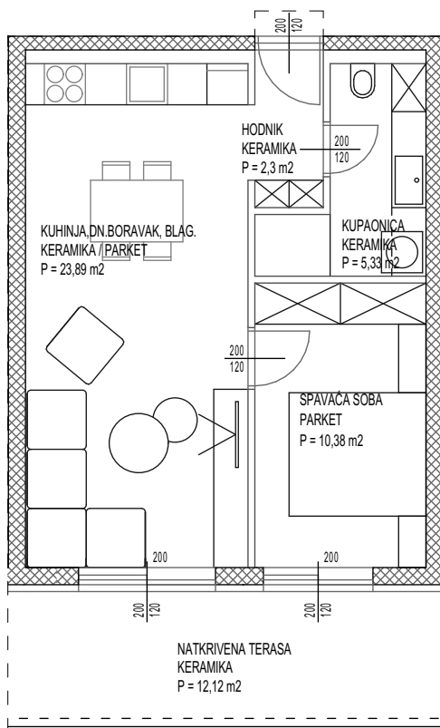
Tlocrt stana
